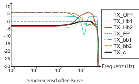
Sendeeigenschaften-Kurve
