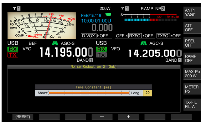
Rauschunterdrückung 2
