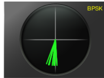
BPSK und QPSK „Ruhe“-Signal
